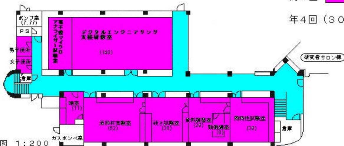
研究棟 1階 平面図 1:200
